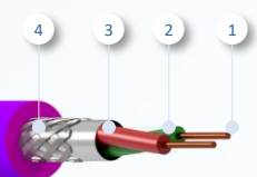
1- Condutor 2- Isolação 3- Blindagem 4- Cobertura
